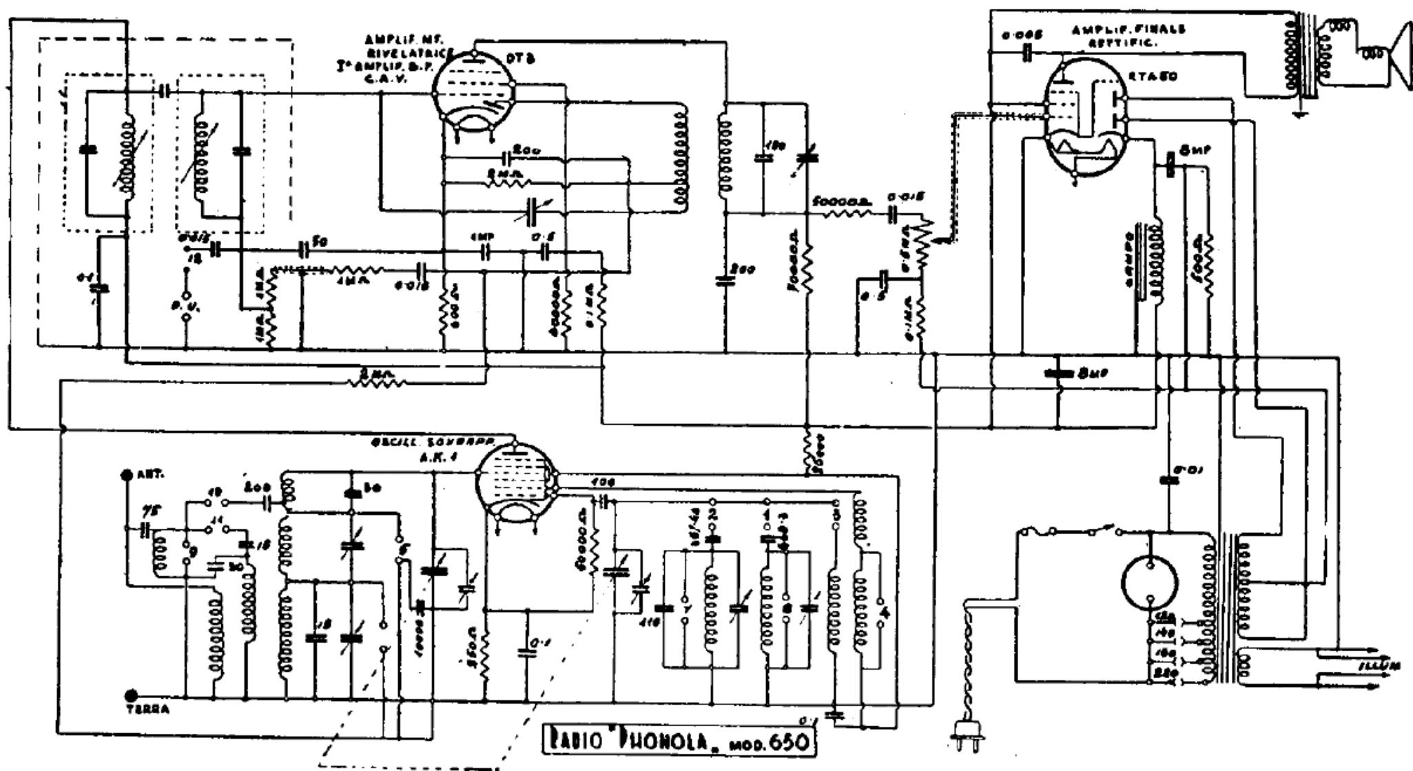
PHONOLA-RADIO (S. A. FIMI). — Modelli: « 650, 651, 652 e 653 ». - Produzione 1934 - Media frequenza: 470 kc.
